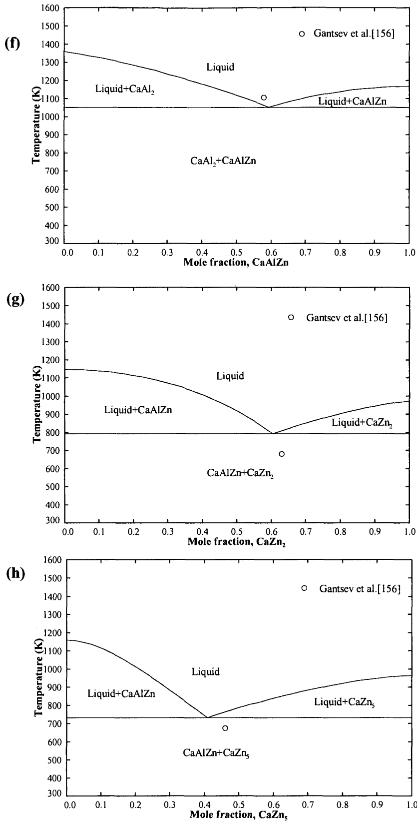
Figure 4.34: Calculated isoplethal analysis of sections (a) Al - AlCaZn , (b) Al - CaZn_{13} , (c) CaAlZn - CaAl_2Zn_2 , (d) CaAlZn - CaZn_{11} , (e) Al_2Ca - CaAl_2Zn_2 , (f) Al_2Ca - CaAlZn , (g) CaAlZn - CaZn_2 , (h) CaAlZn - CaZn_5
