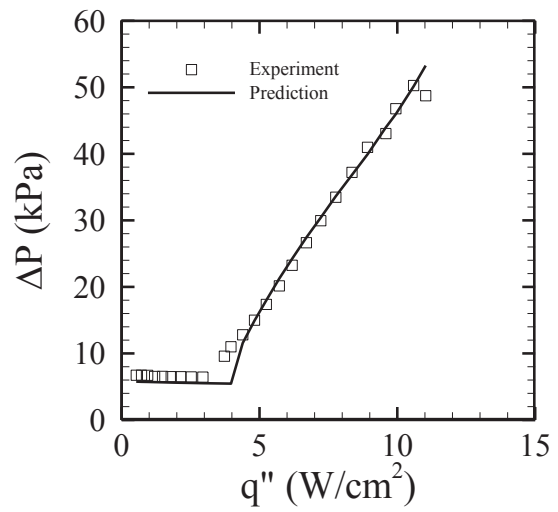
(d) G = 550 \text{ kg/m}^2\cdot\text{s}
