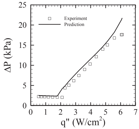
(b) G = 295 \text{ kg/m}^2\cdot\text{s}
